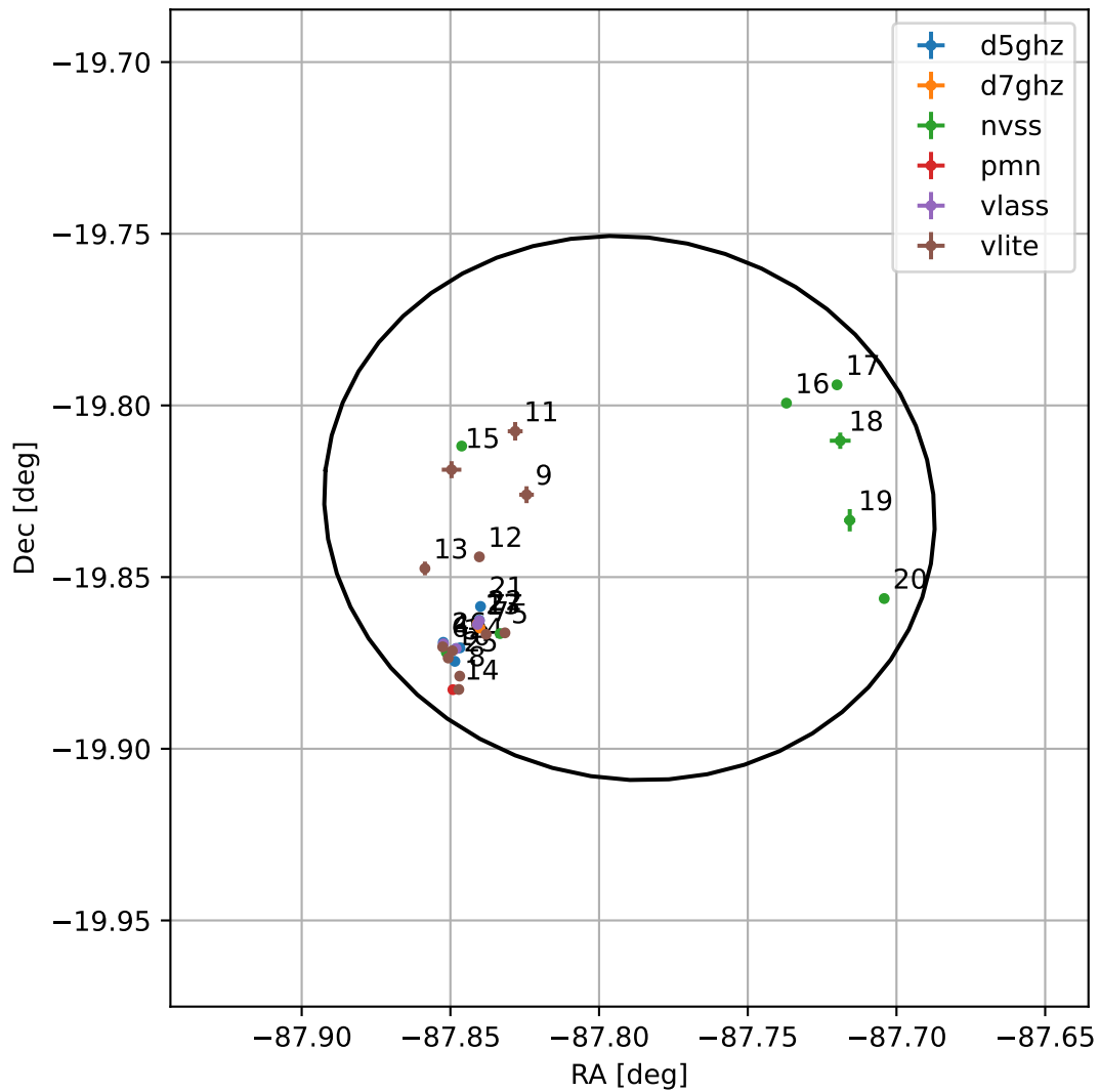
4FGL J1808.8-1949
