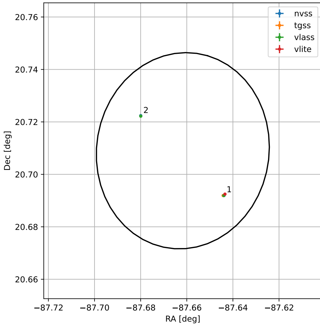
4FGL J1809.3+2042
