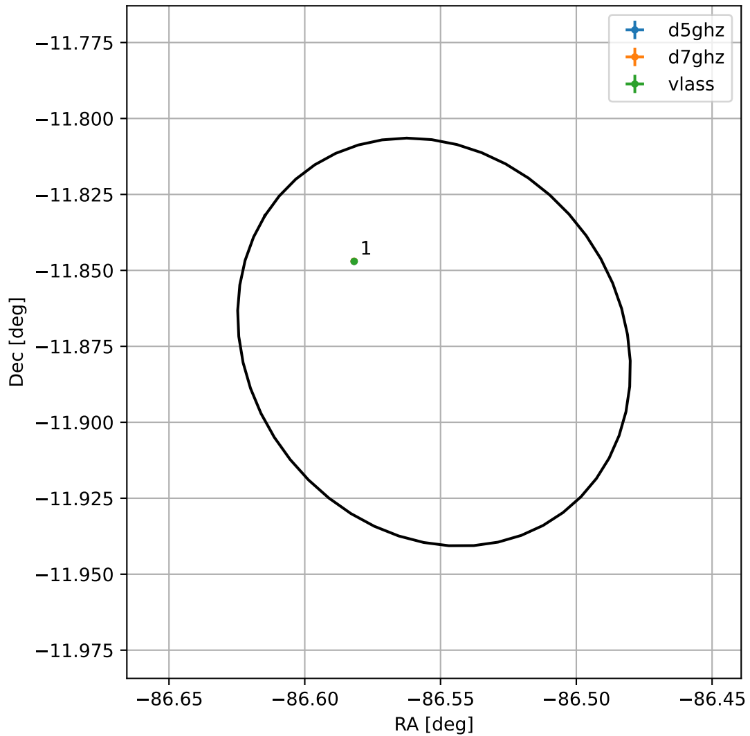
4FGL J1813.7-1152
