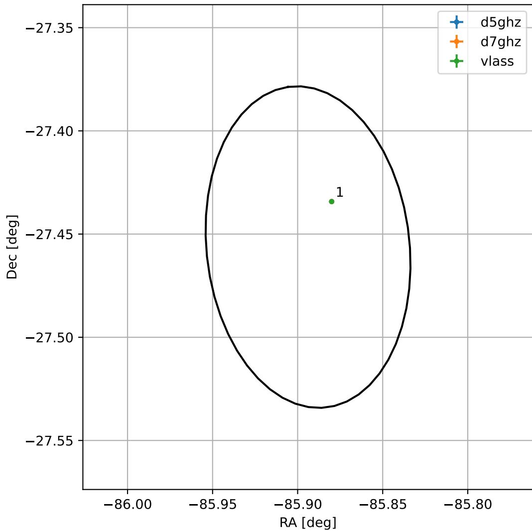
4FGL J1816.4-2727
