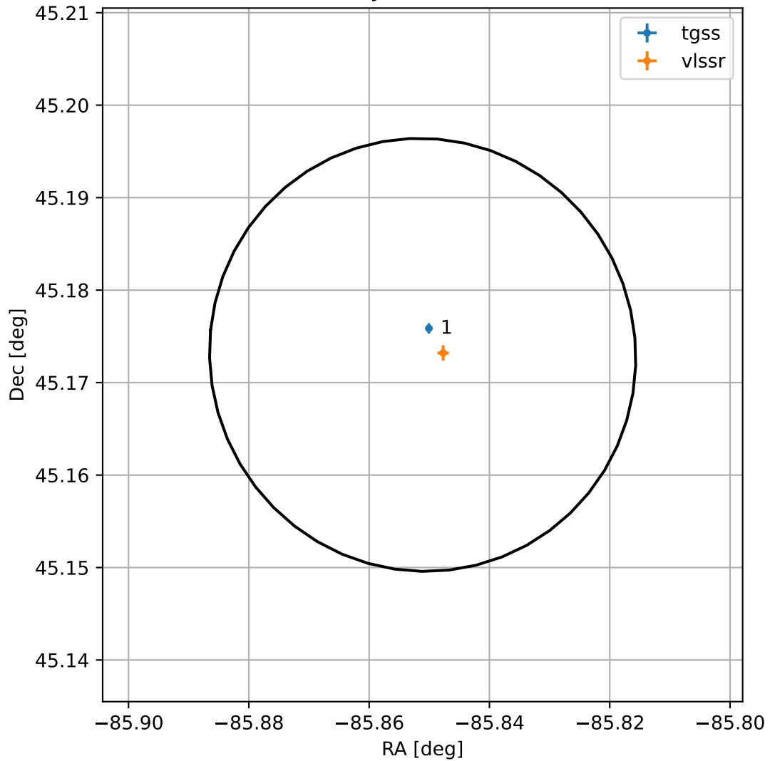
4FGL J1816.5+4510
