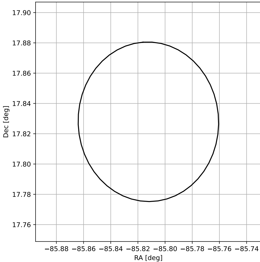
4FGL J1816.7+1749
