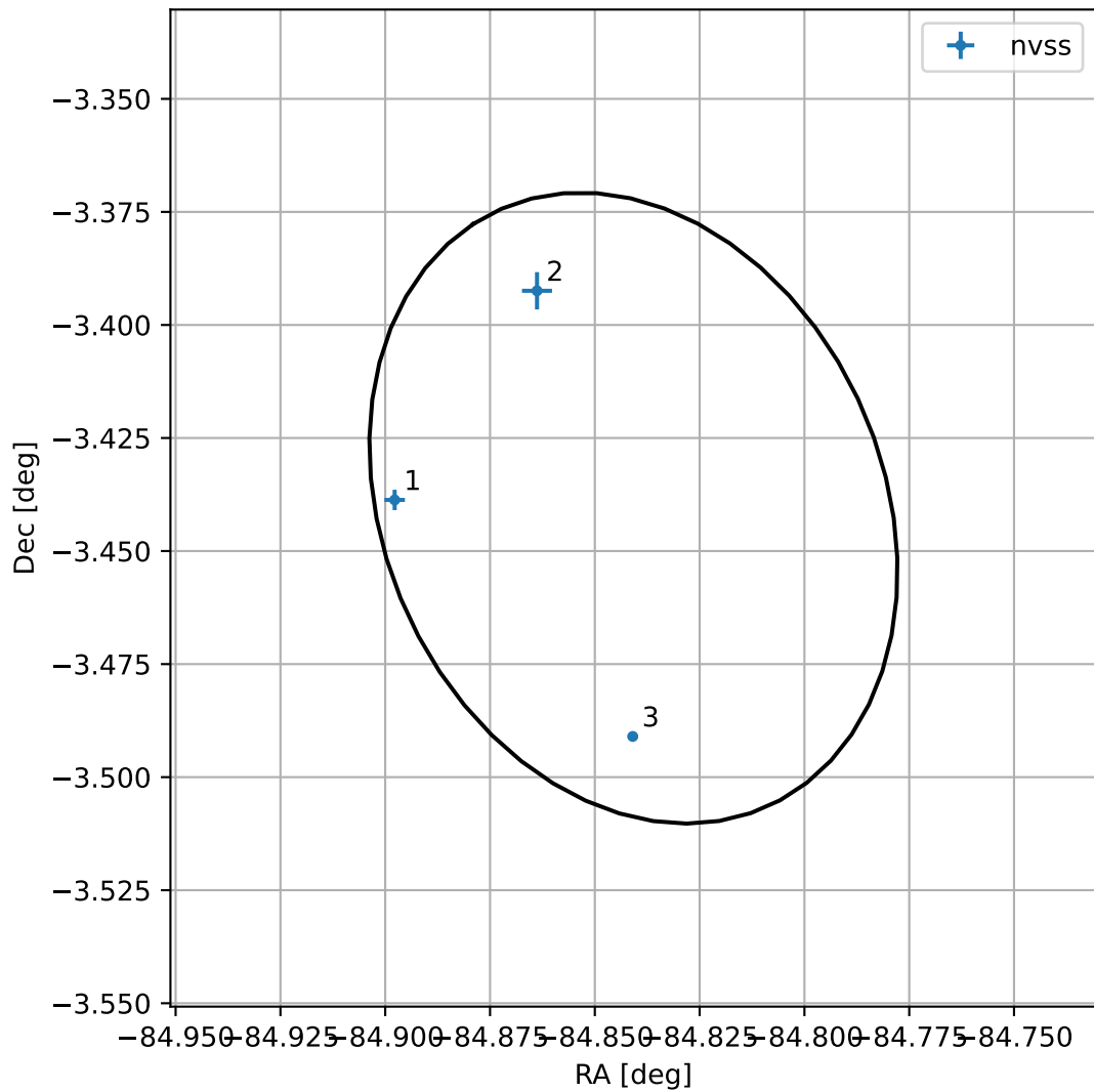
4FGL J1820.6-0326
