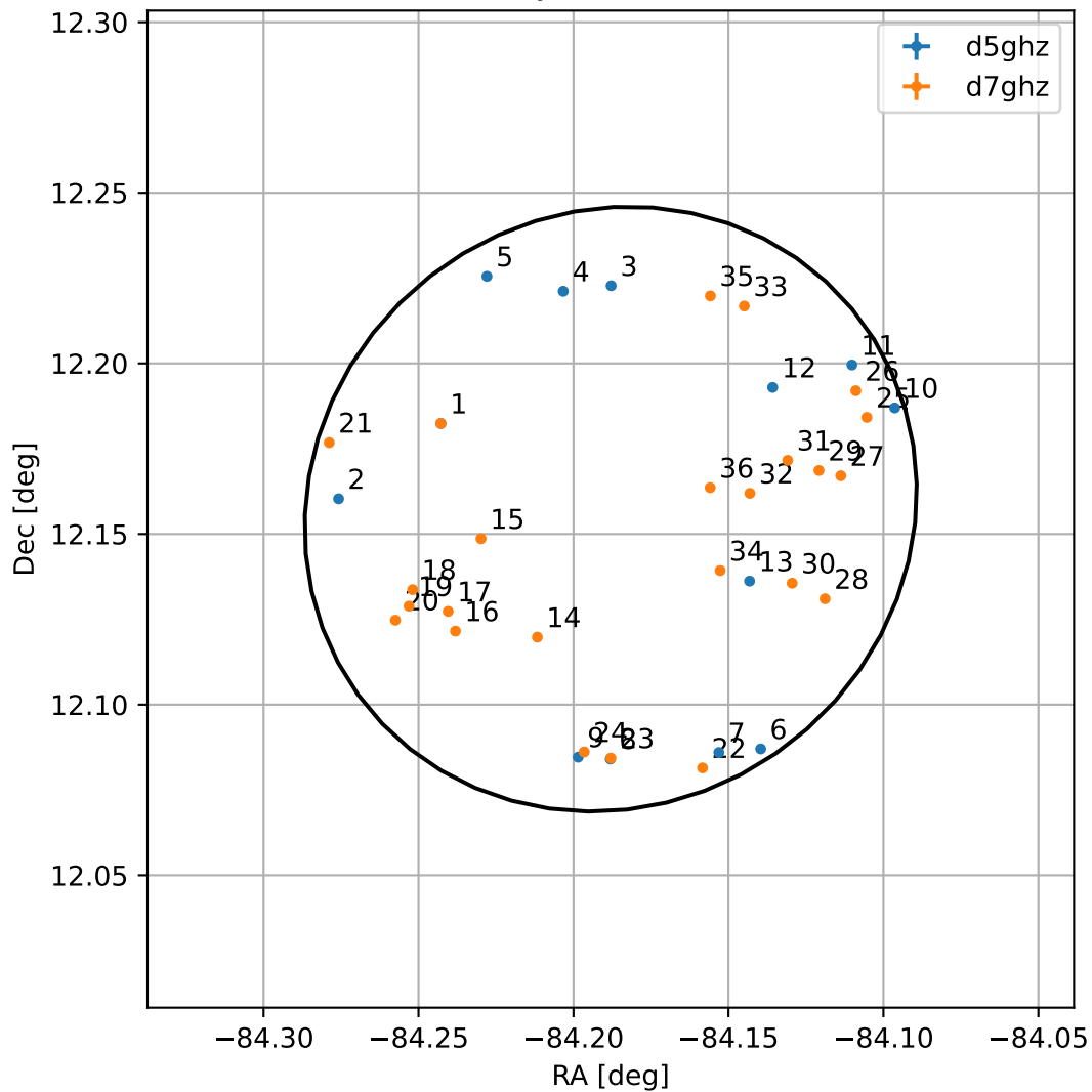
4FGL J1823.2+1209
