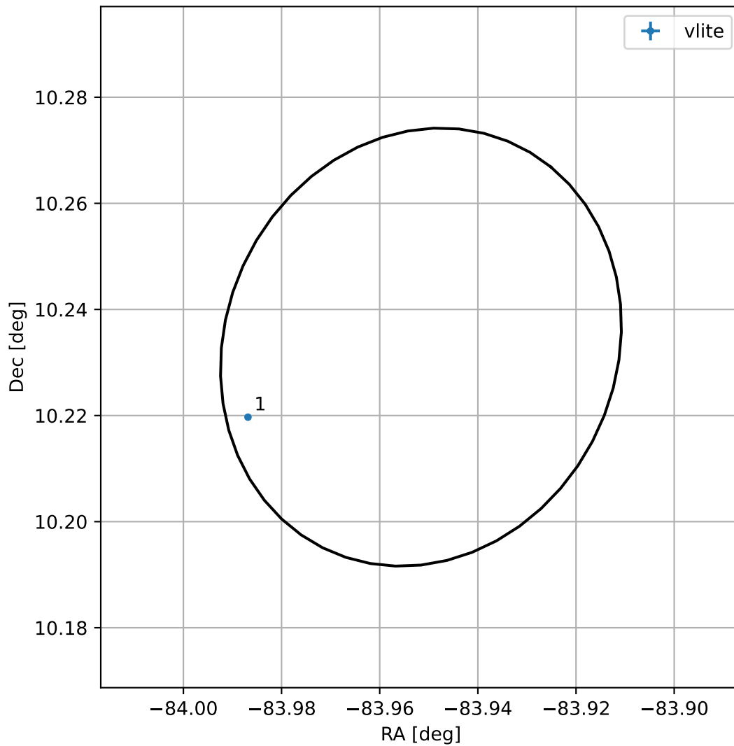
4FGL J1824.1+1013
