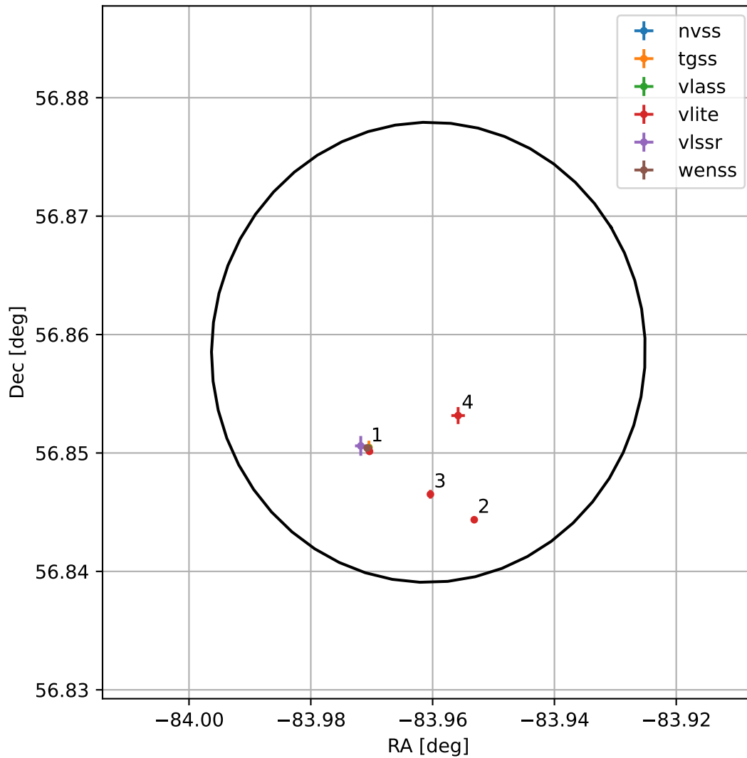
4FGL J1824.1+5651
