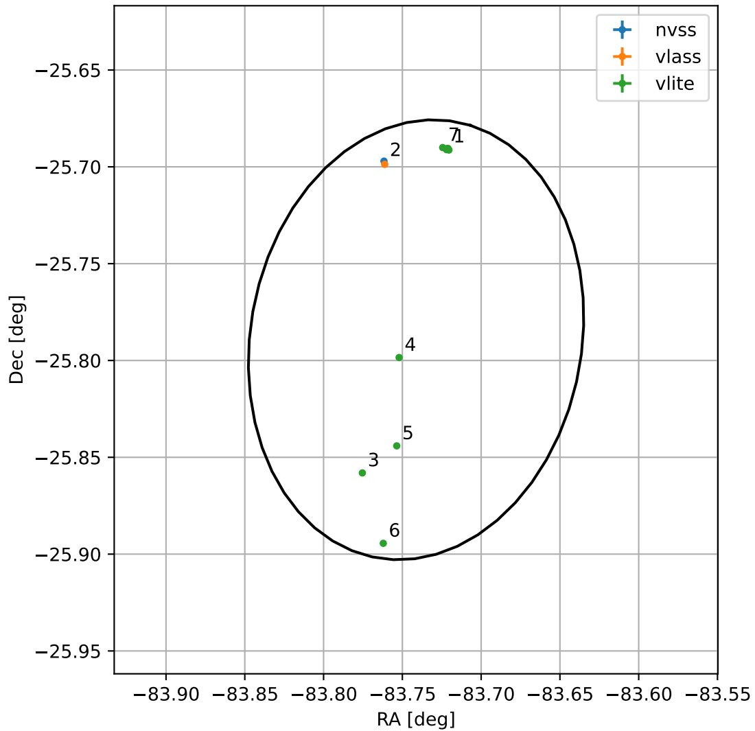
4FGL J1825.0-2547
