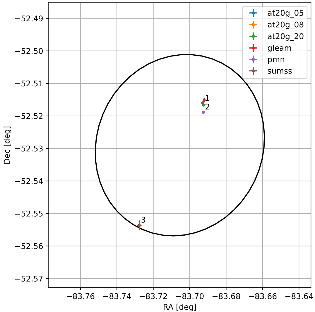
4FGL J1825.1-5231
