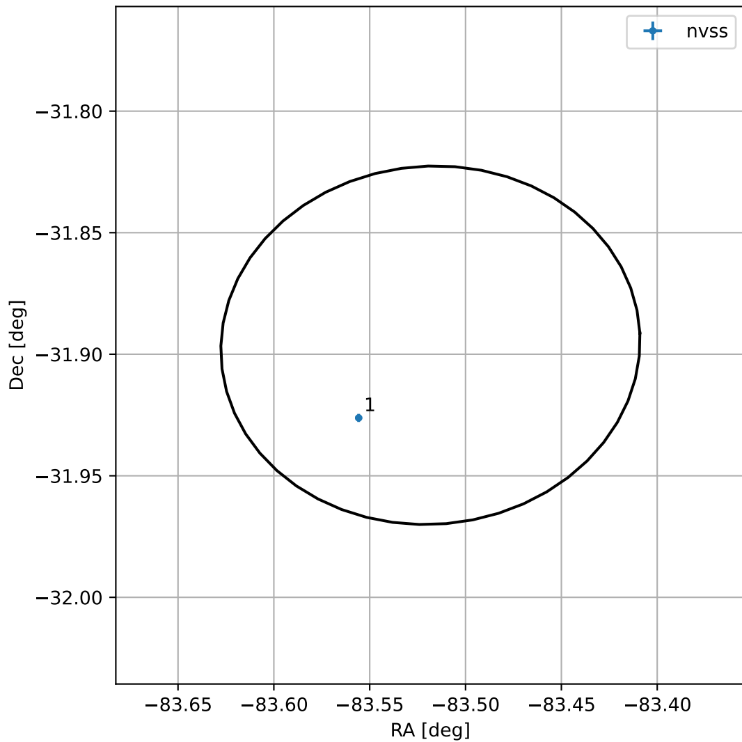
4FGL J1825.9-3153
