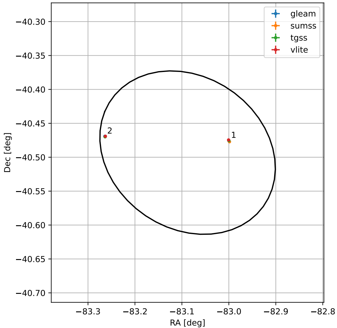
4FGL J1827.6-4029
