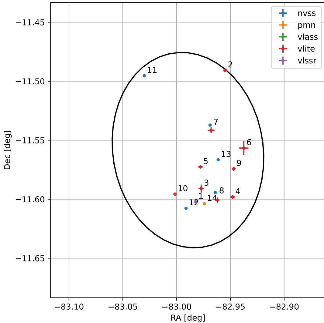
4FGL J1828.0-1133
