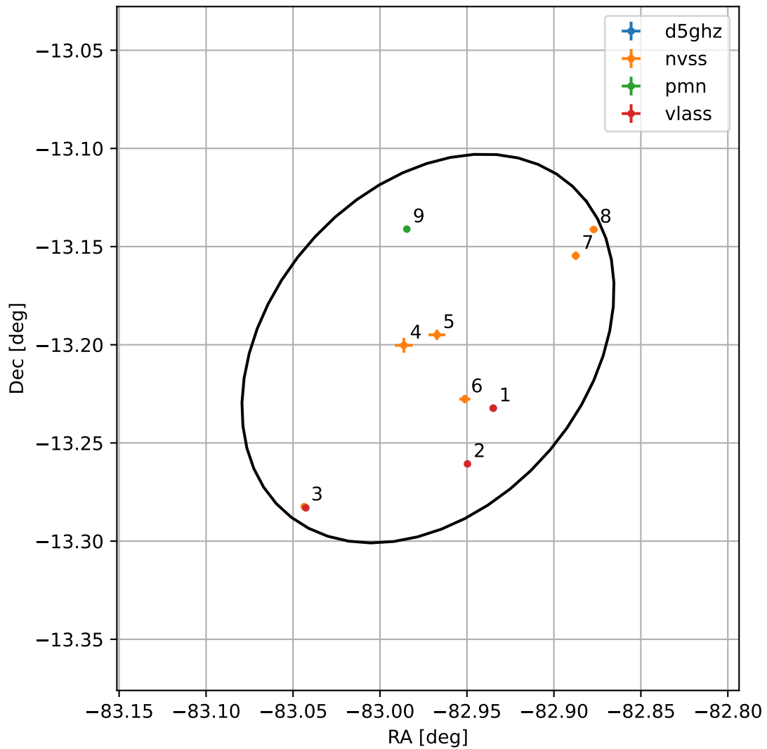
4FGL J1828.1-1312
