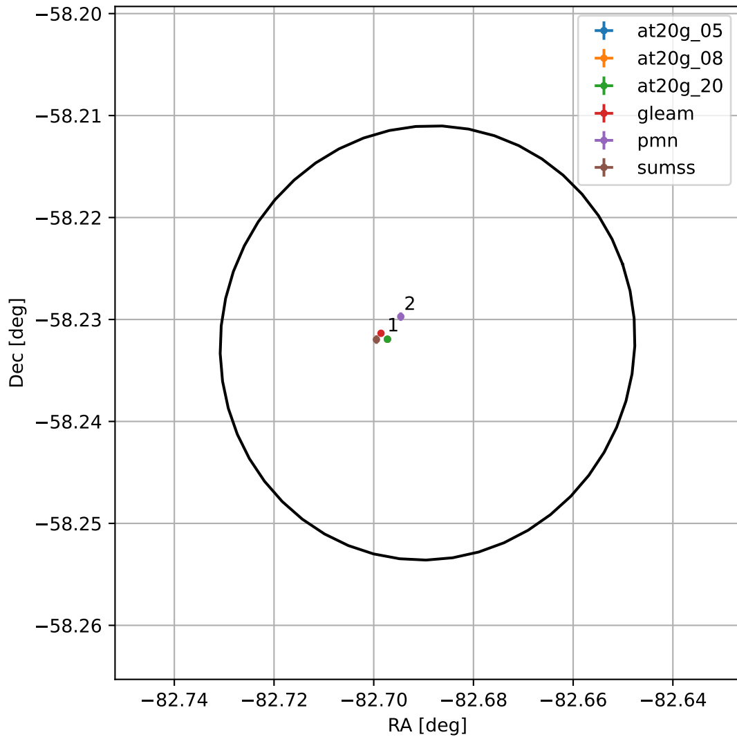
4FGL J1829.2-5813
