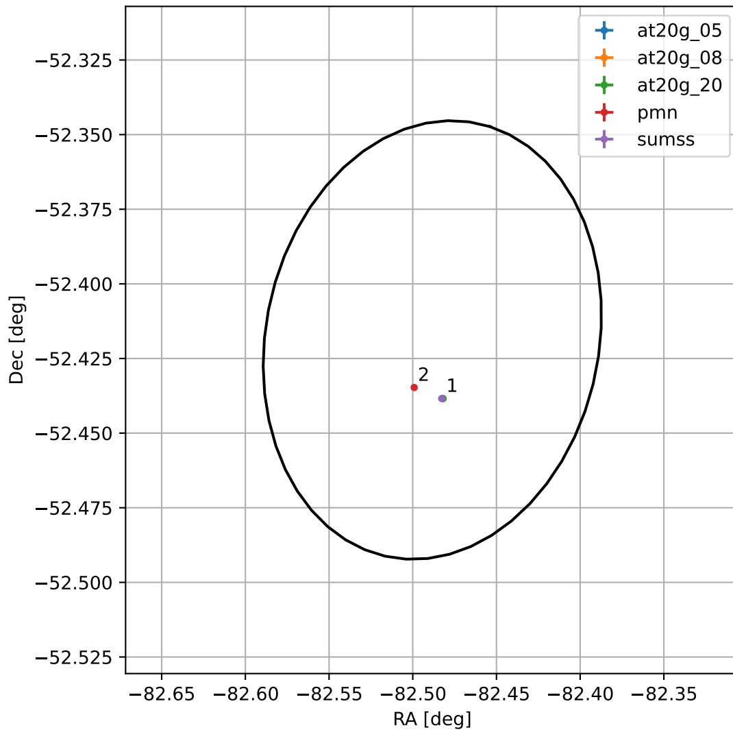
4FGL J1830.0-5225
