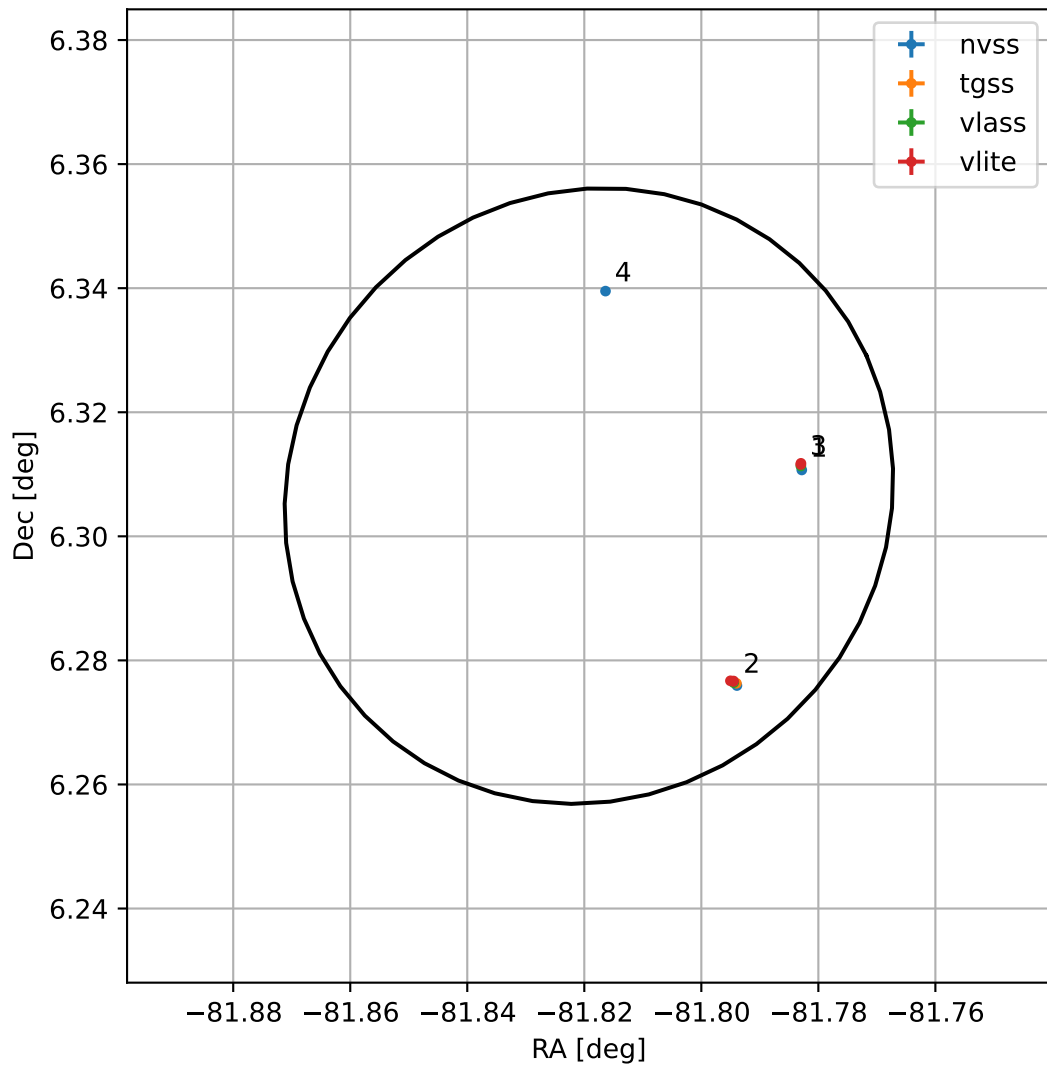
4FGL J1832.7+0618
