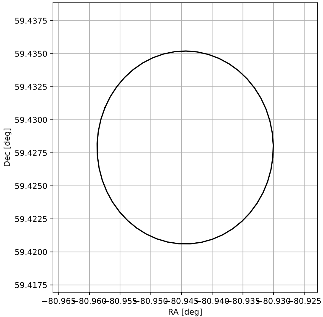
4FGL J1836.2+5925
