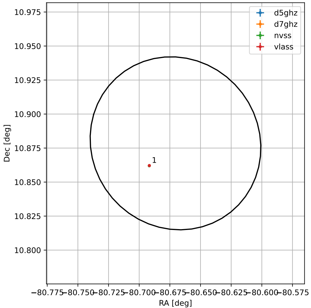
4FGL J1837.3+1052
