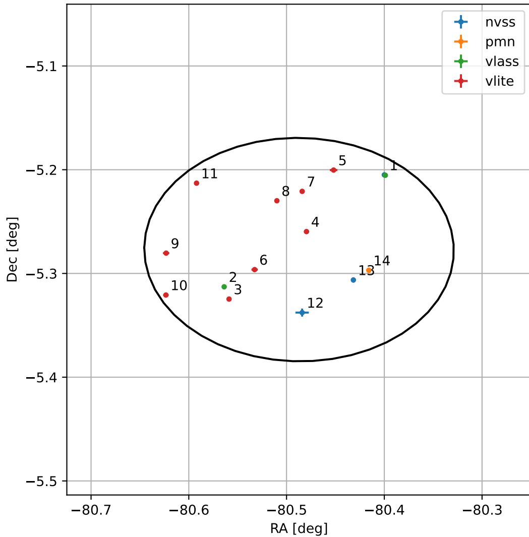
4FGL J1838.0-0516
