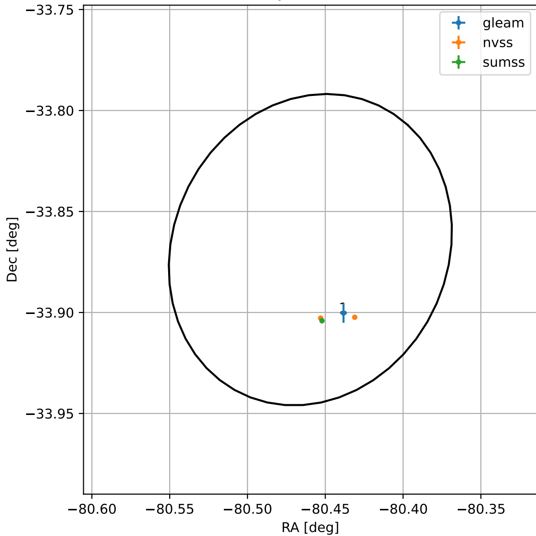
4FGL J1838.1-3352
