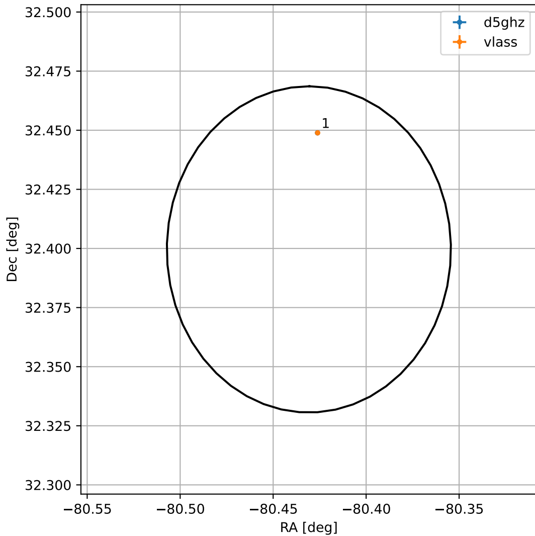
4FGL J1838.2+3223
