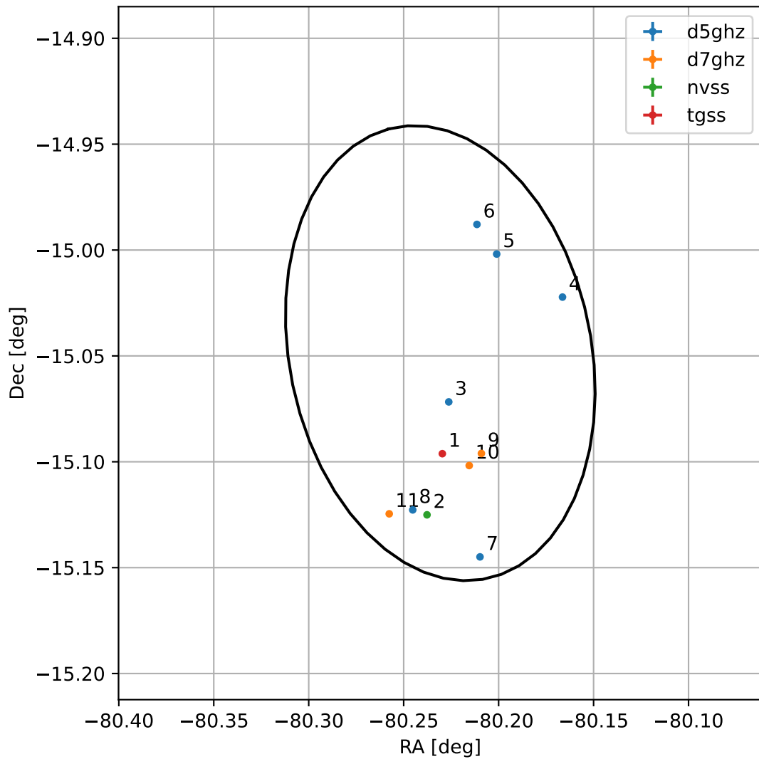
4FGL J1839.0-1502
