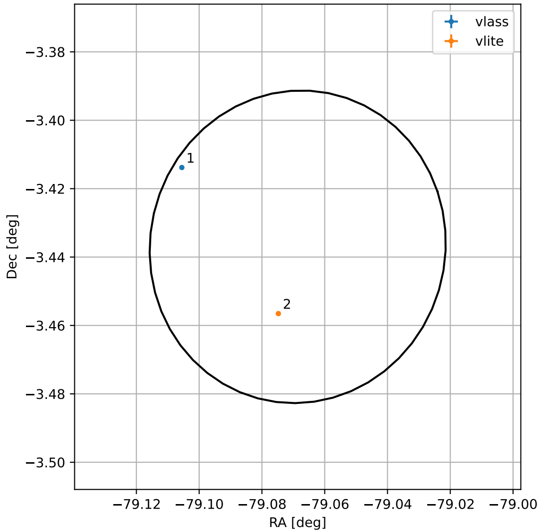
4FGL J1843.7-0326
