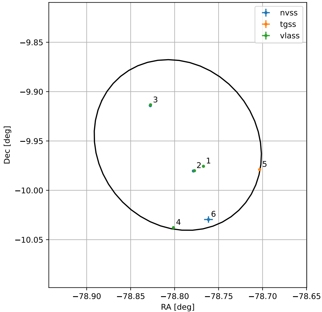
4FGL J1844.8-0957
