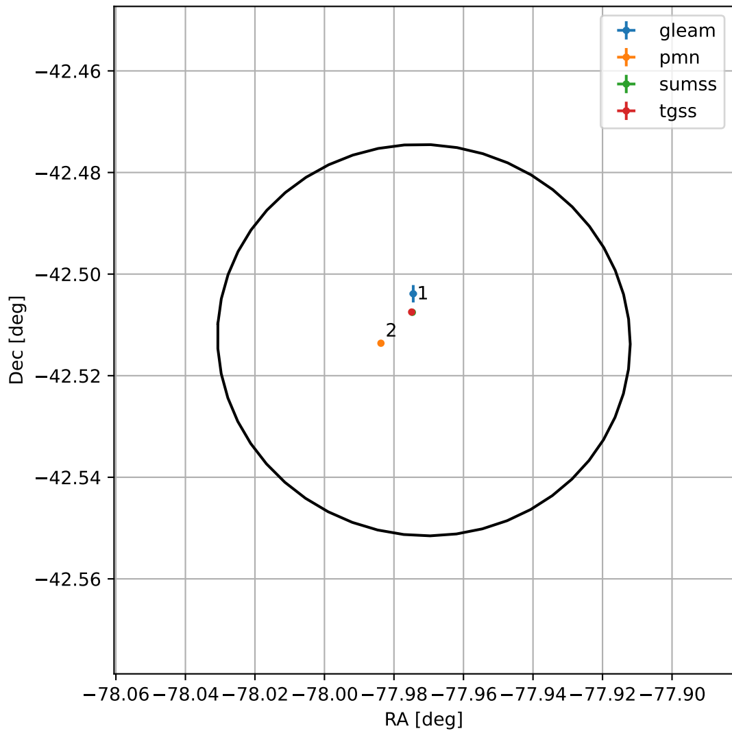
4FGL J1848.1-4230
