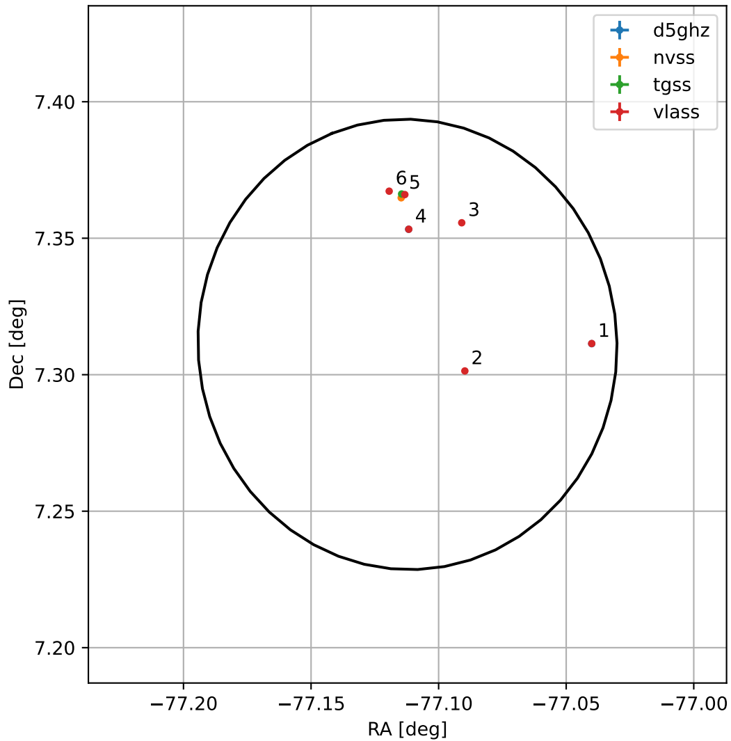
4FGL J1851.5+0718
