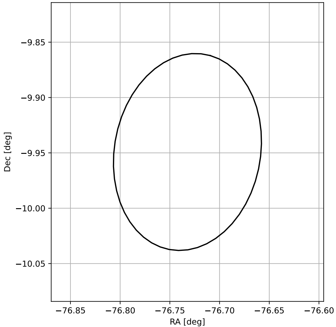
4FGL J1853.0-0956
