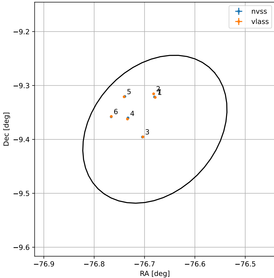
4FGL J1853.2-0922
