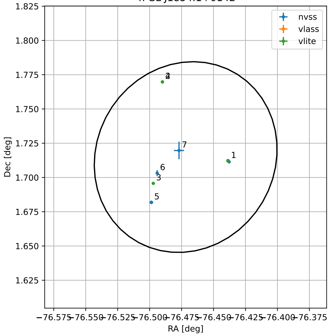
4FGL J1854.1+0142
