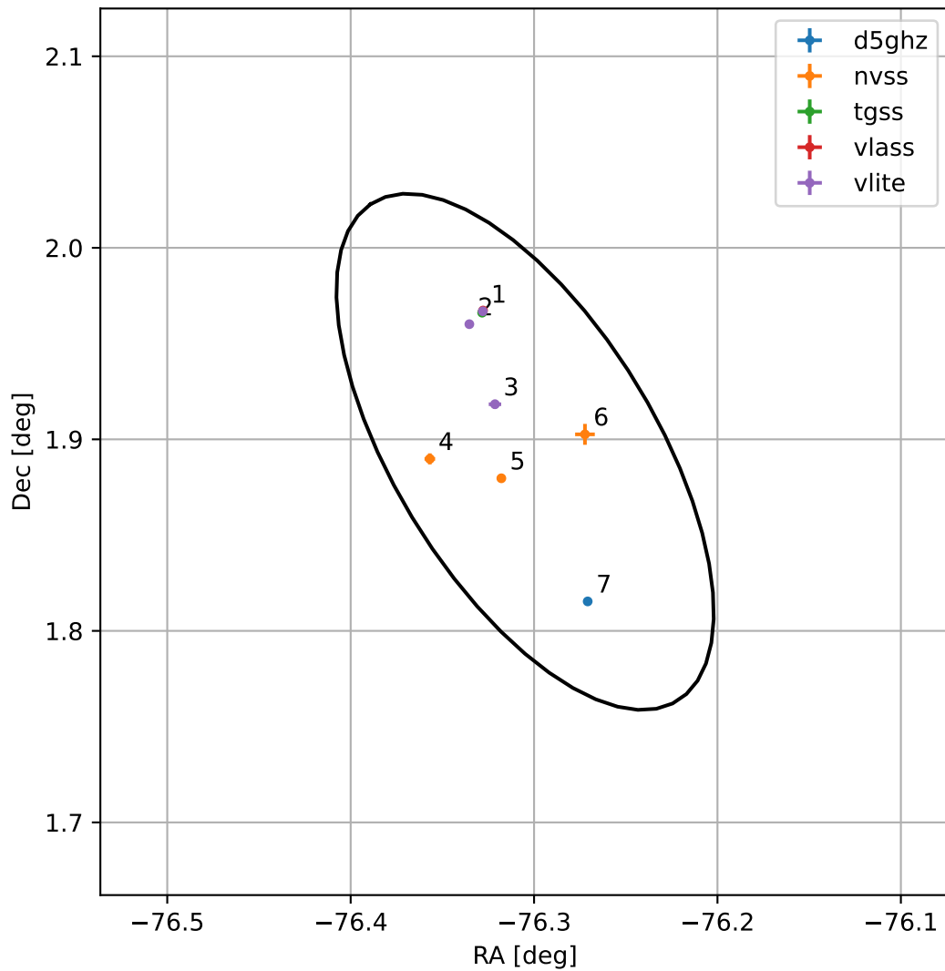
4FGL J1854.7+0153
