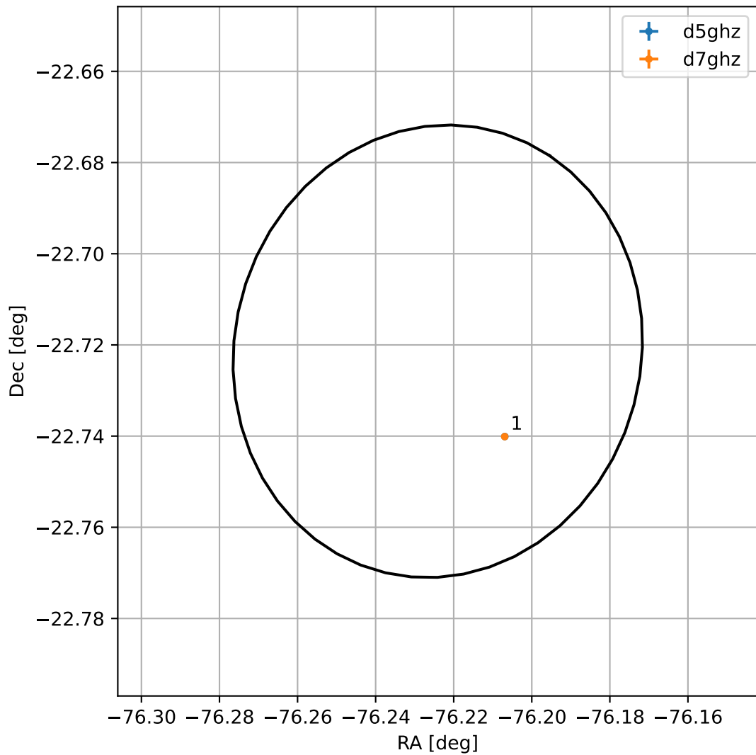
4FGL J1855.1-2243
