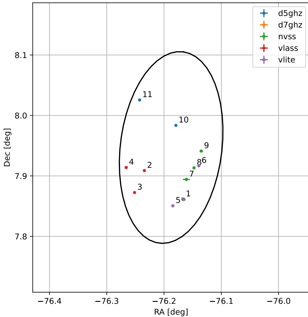
4FGL J1855.2+0756
