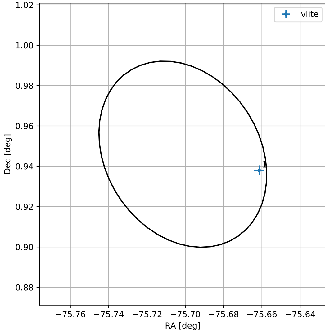
4FGL J1857.1+0056
