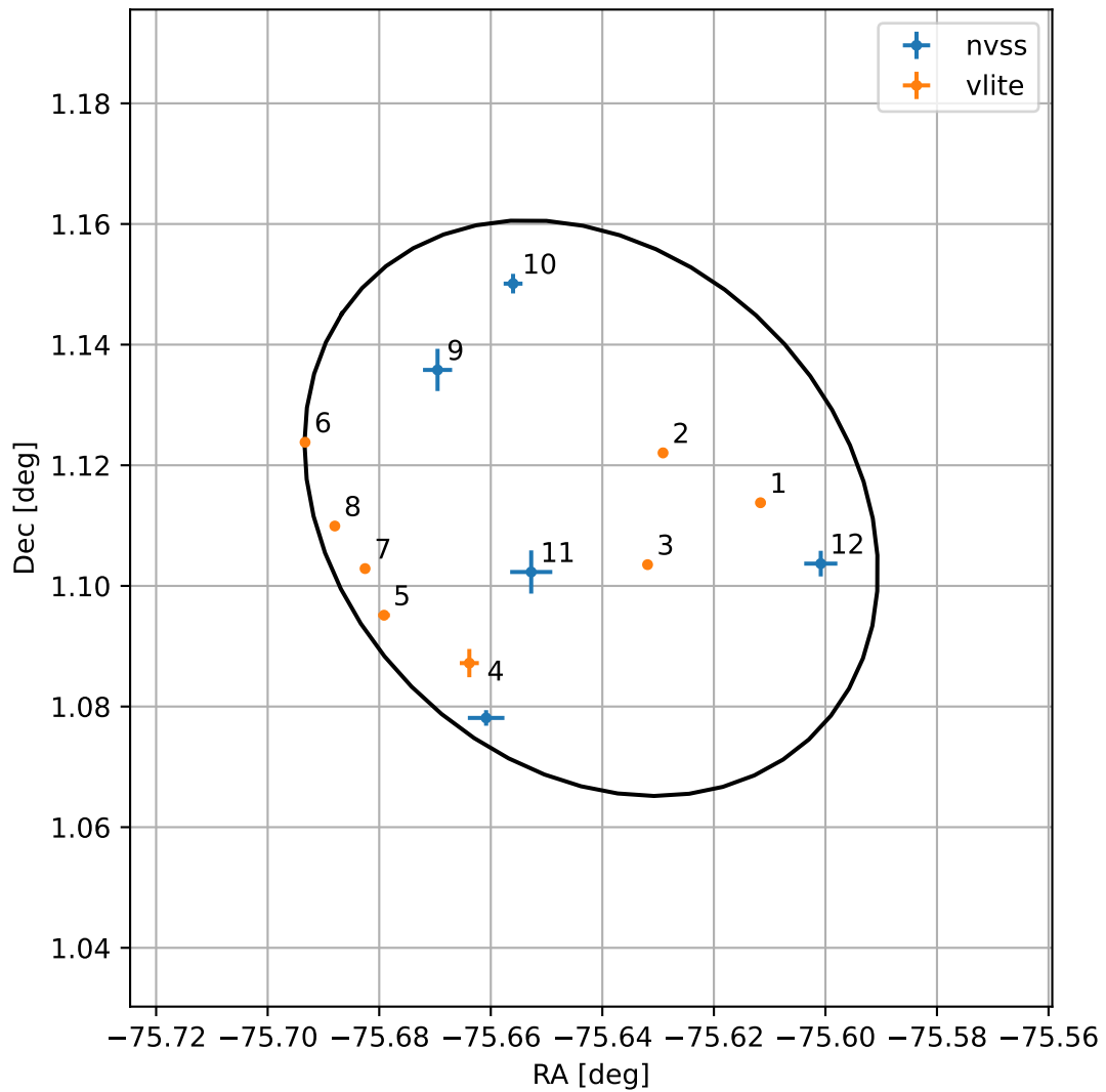
4FGL J1857.4+0106
