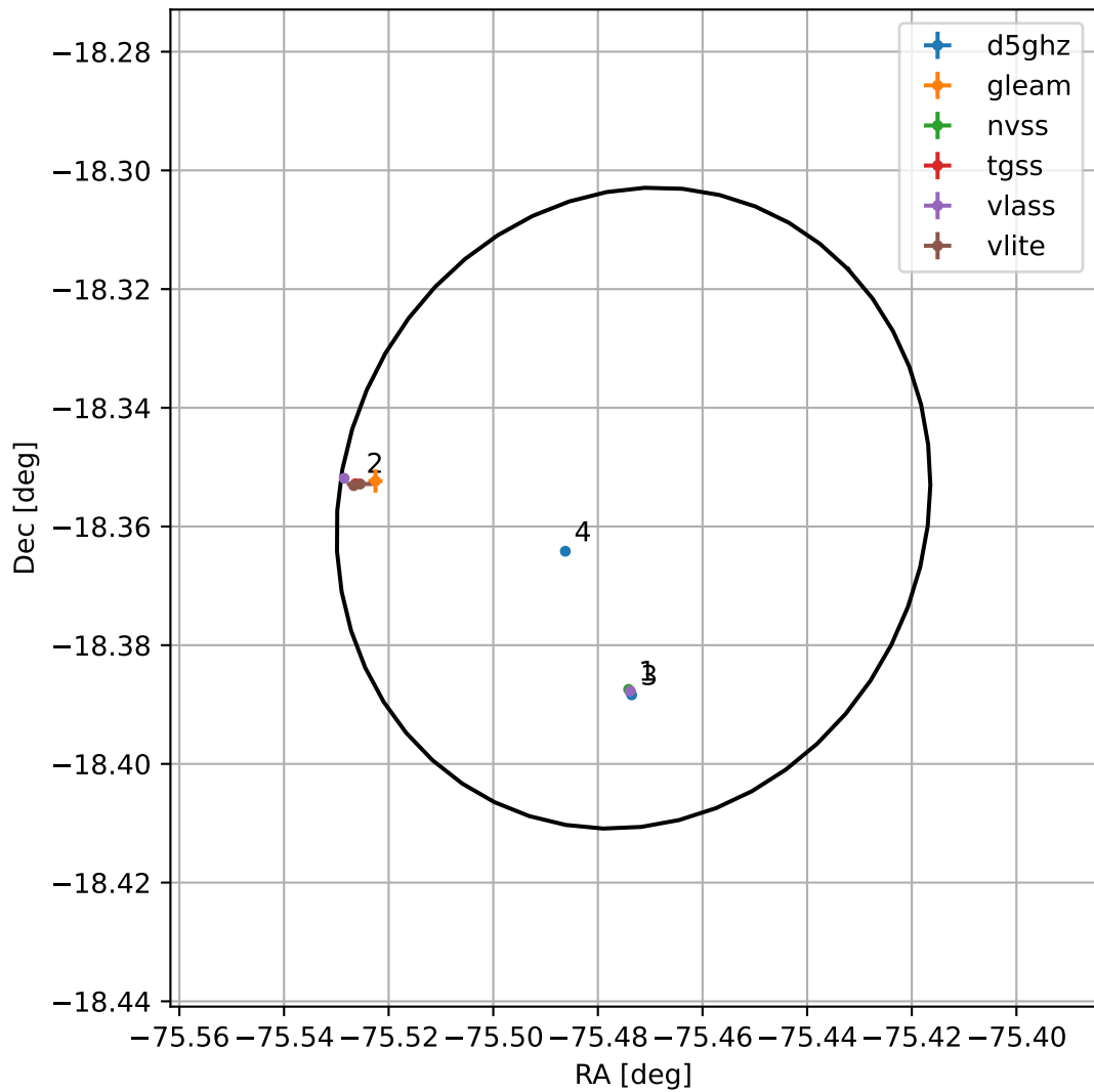
4FGL J1858.1-1821
