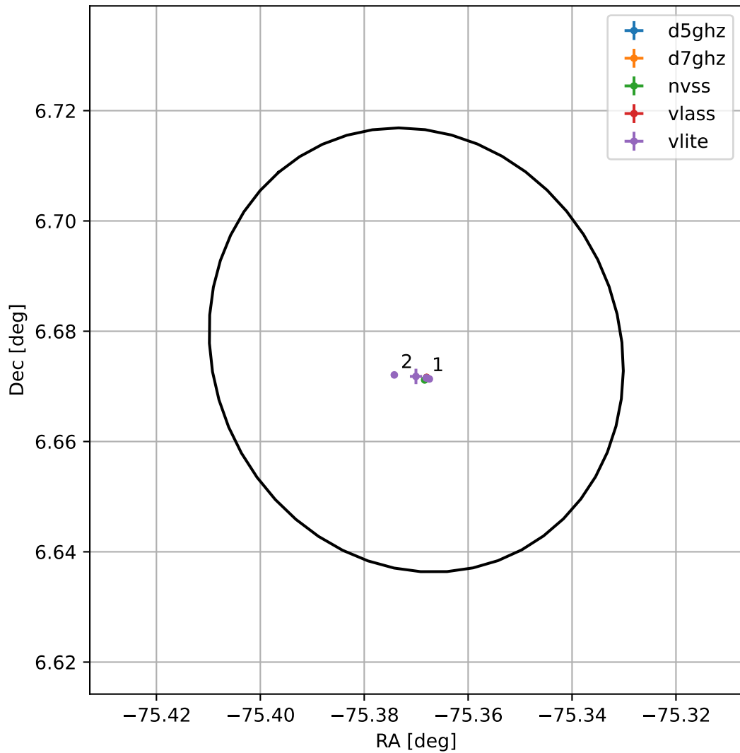
4FGL J1858.5+0640
