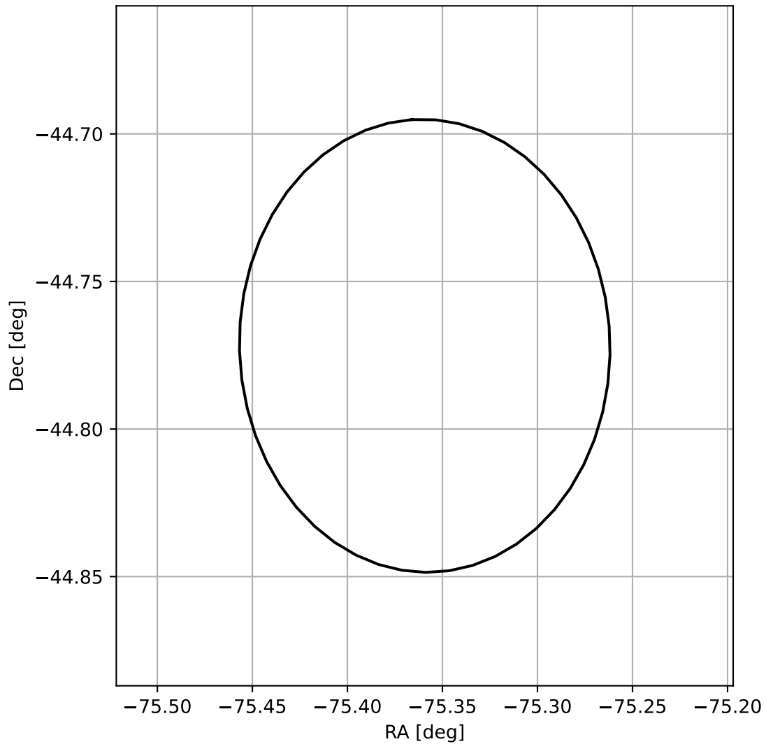
4FGL J1858.5-4446
