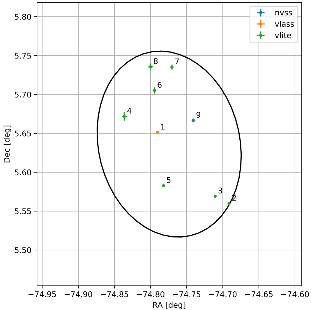
4FGL J1900.9+0538
