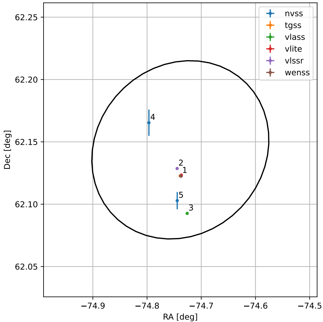
4FGL J1901.0+6208
