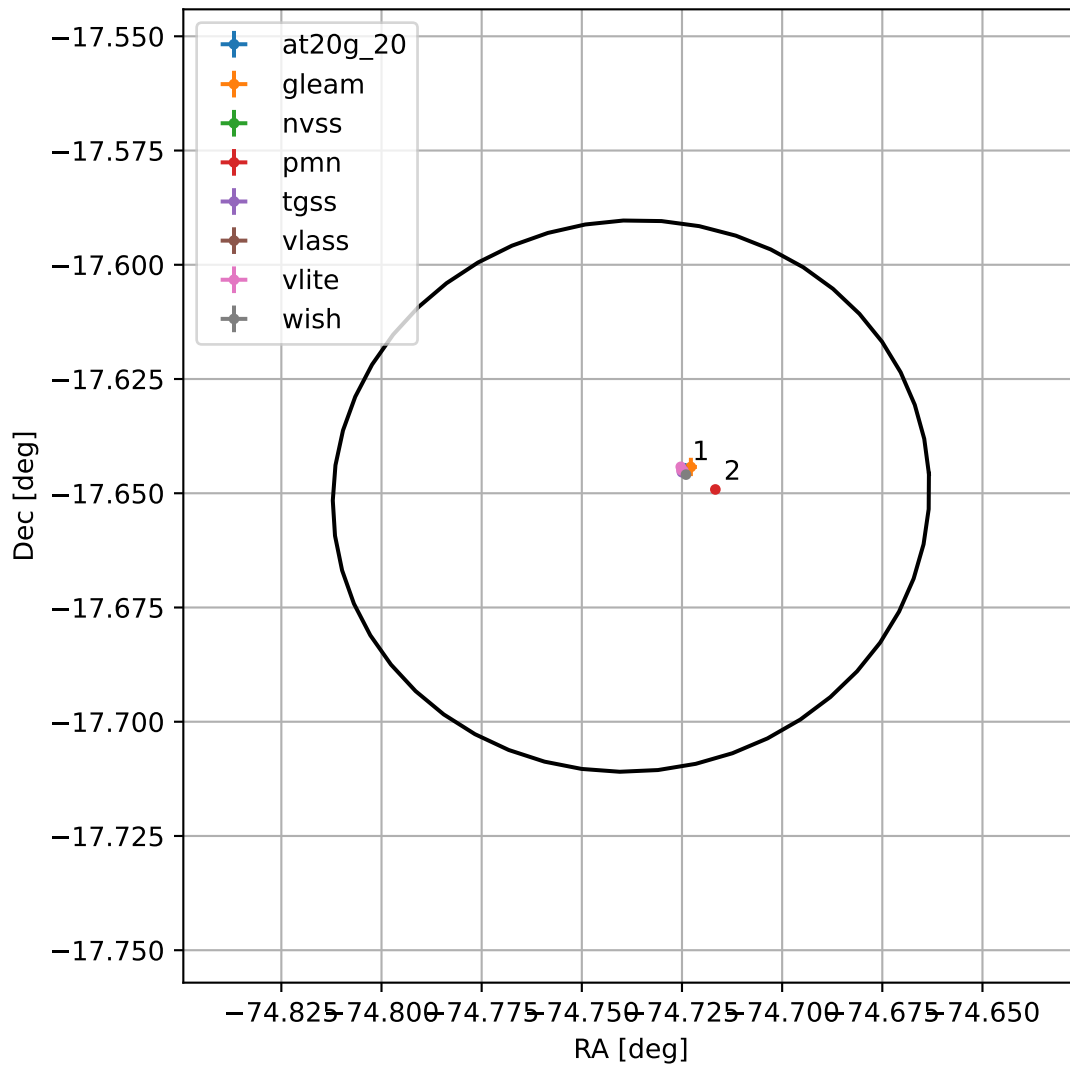
4FGL J1901.0-1739
