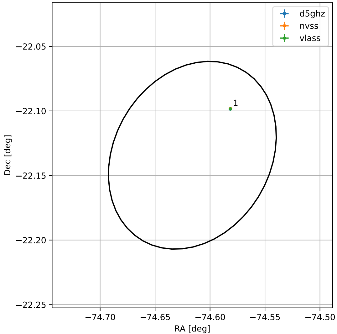
4FGL J1901.5-2208
