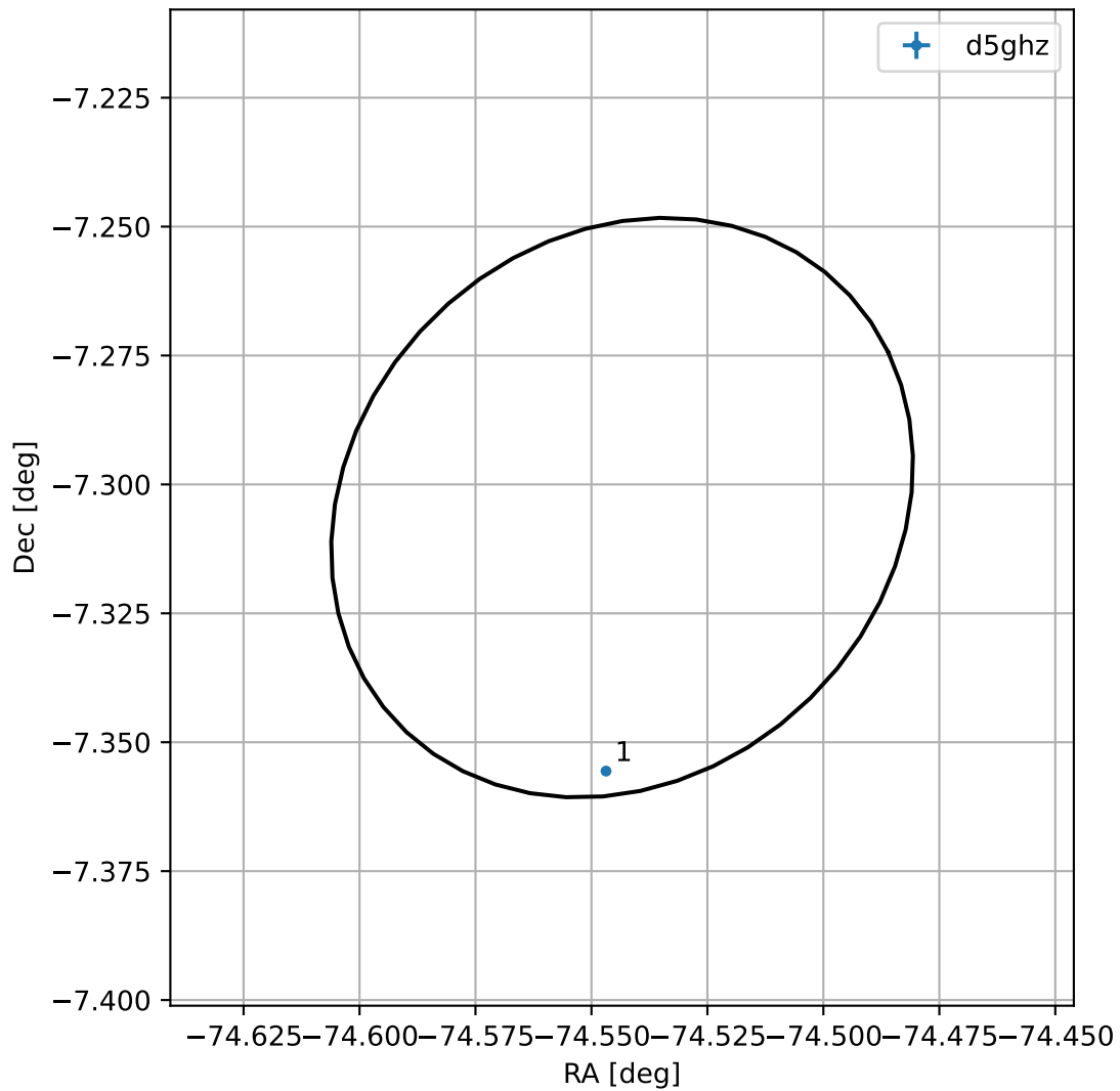
4FGL J1901.8-0718
