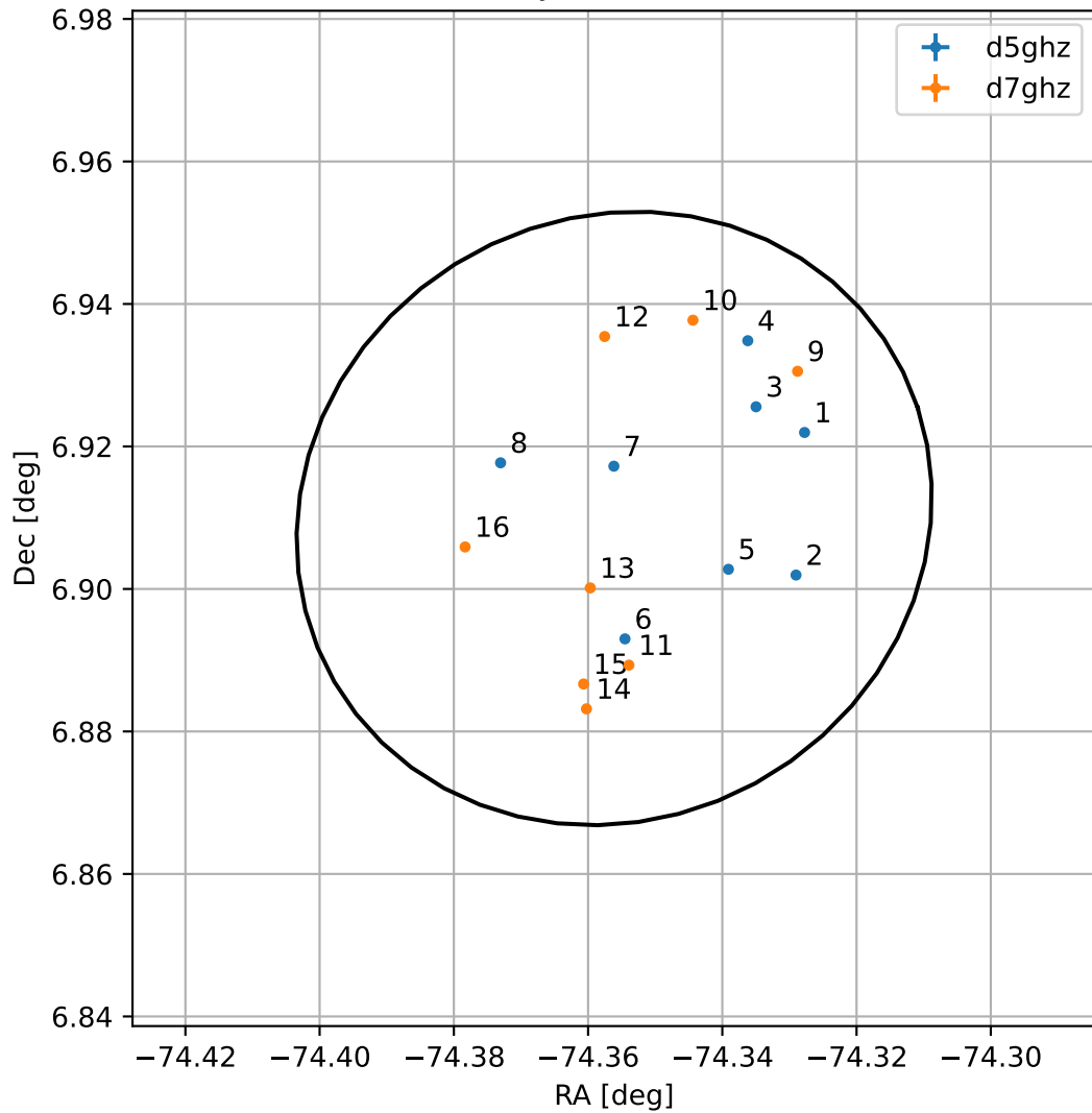
4FGL J1902.5+0654
