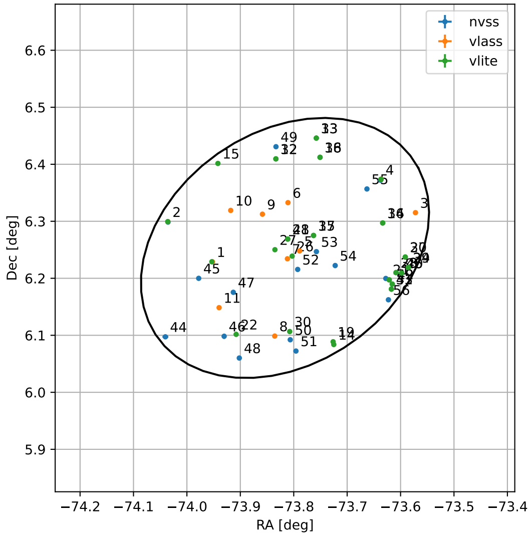
4FGL J1904.7+0615
