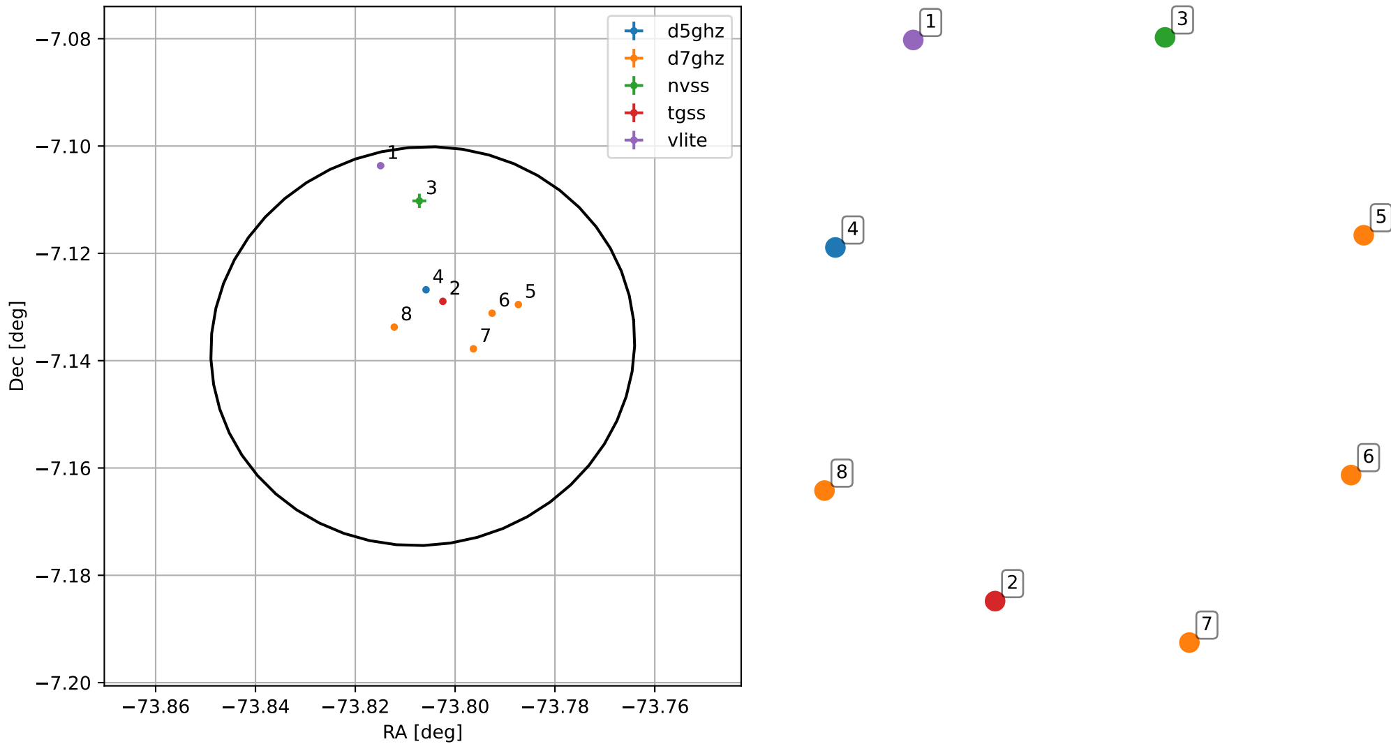
4FGL J1904.7-0708
