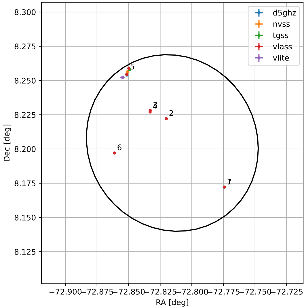
4FGL J1908.7+0812
