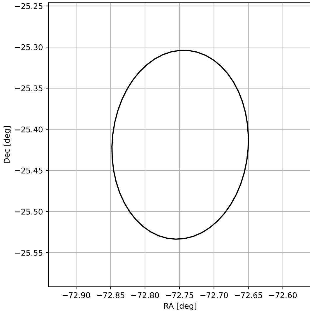
4FGL J1909.0-2525
